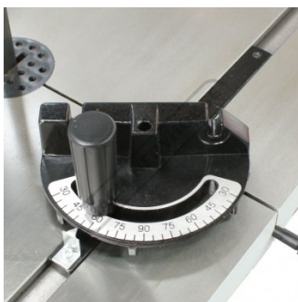
Mitre Guide
